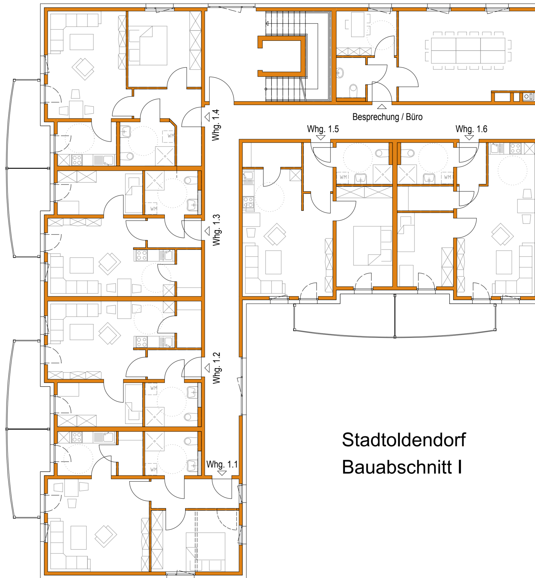
1. Obergeschoss
